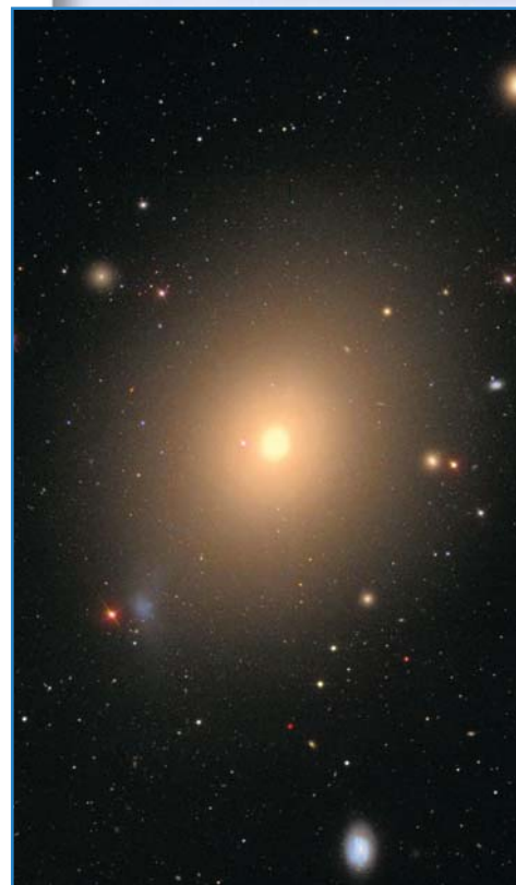
Эллиптическая галактика М49 в созвездии Девы
