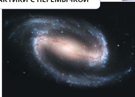
СПИРАЛЬНЫЕ ГАЛАКТИКИ С ПЕРЕМЫЧКОЙ
