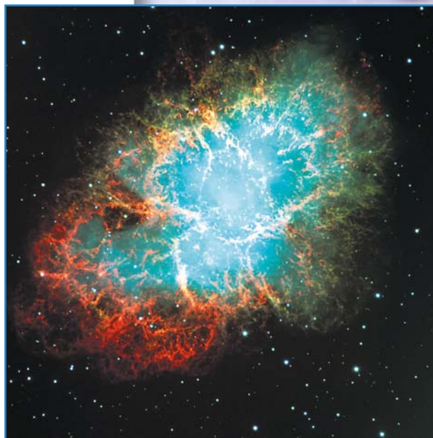
Крабовидная туманность — остаток взрыва сверхновой звезды
