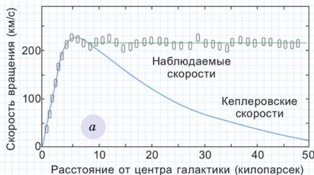
Скорость вращения галактики на различных расстояниях от центра
