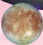
Европа
