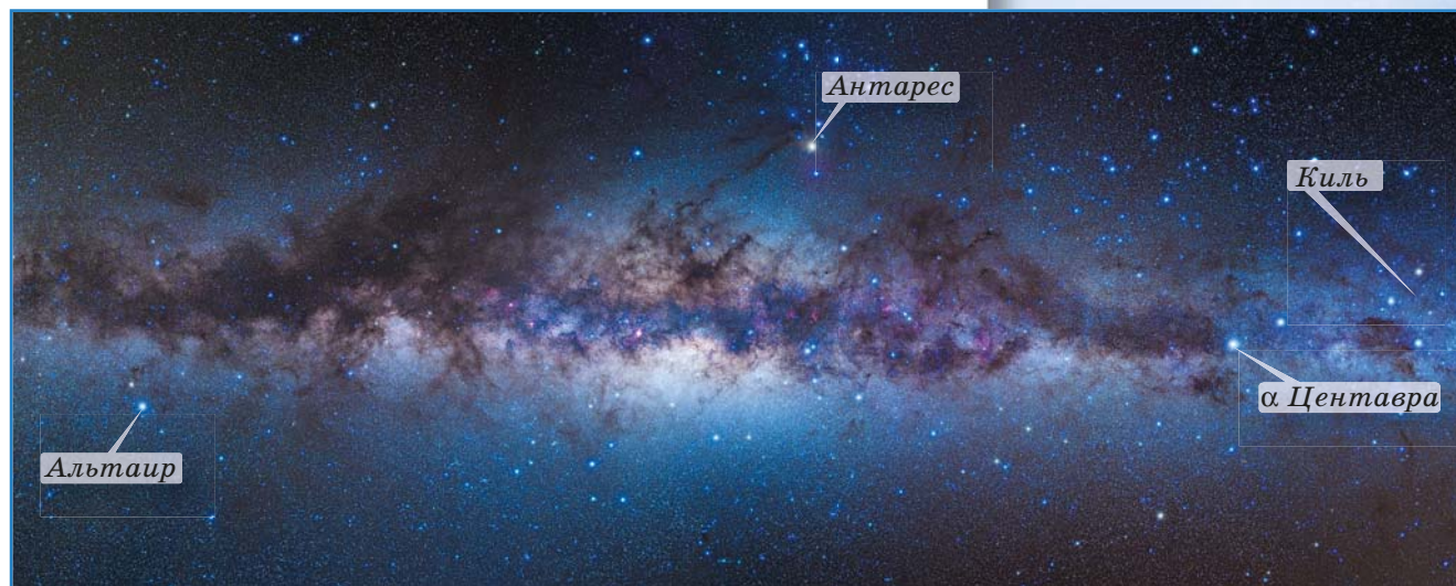
Часть Млечного Пути от созвездия Орла до созвездия Кита
