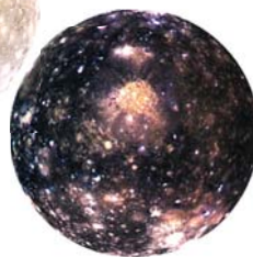
Каллисто
