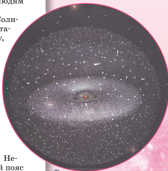
Облако Оорта
