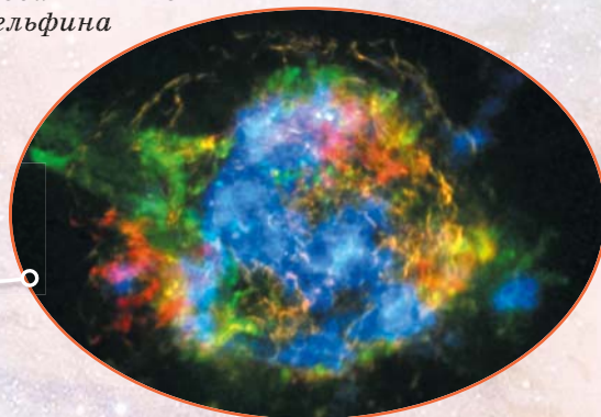
Вспышка новой звезды в созвездии Дельфина
