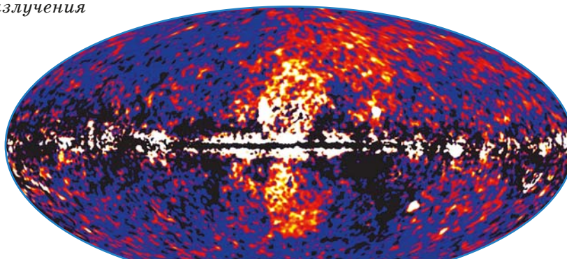
Карта распределения \gamma -излучения
