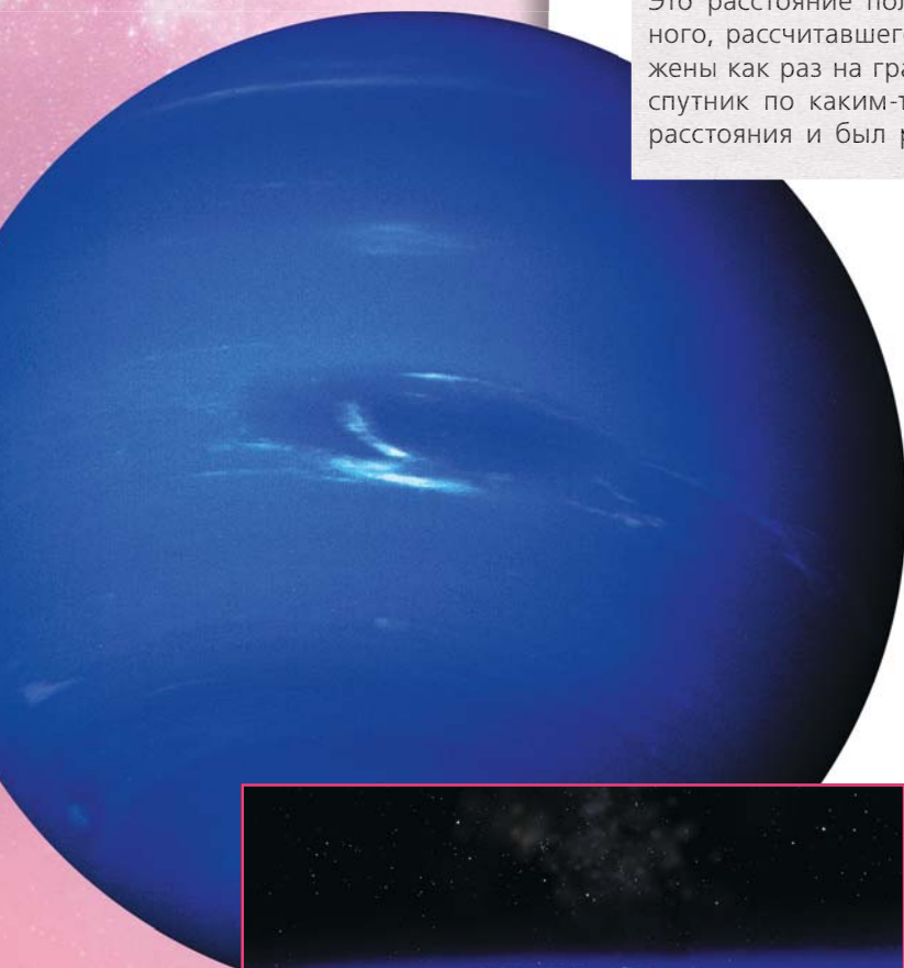
Нептун
