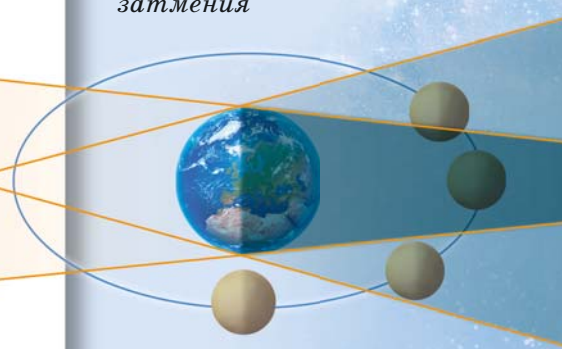
Схема лунного затмения
