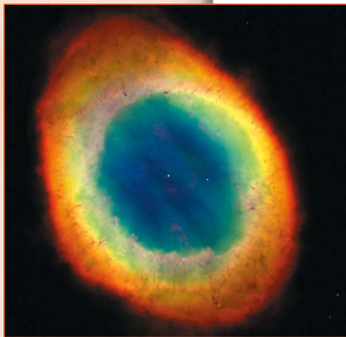
Планетарная туманность M57 «Кольцо» в созвездии Лиры
