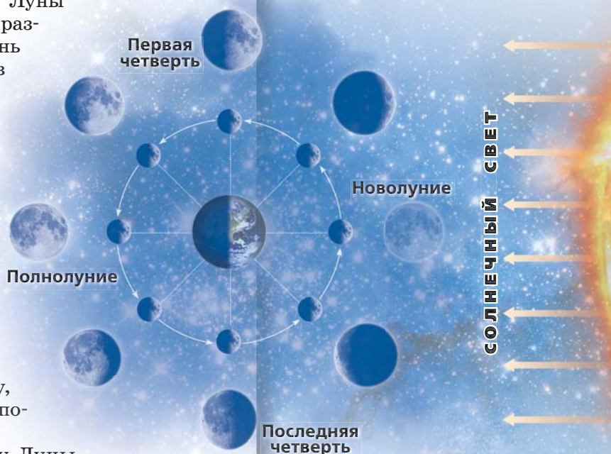
Фазы Луны
